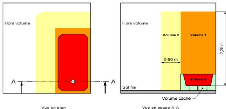
Figure 701B - Exemple de local contenant une baignoire ou une douche avec receveur
